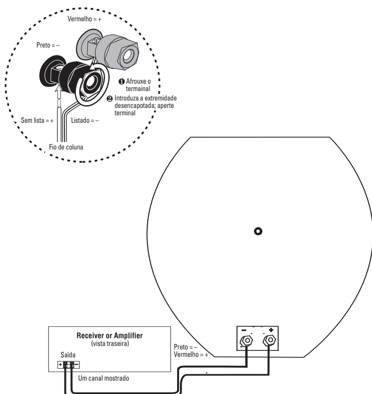
Figura 3. O diagrama da cablagem apresenta a polaridade das ligações relativamente a um dos canais de um sistema de cinema em casa.
